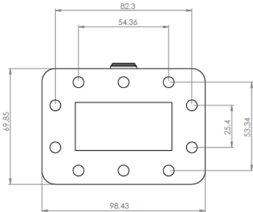
UDR40 Flange
