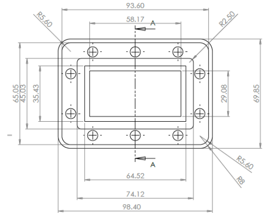
CPRG40 Flange
